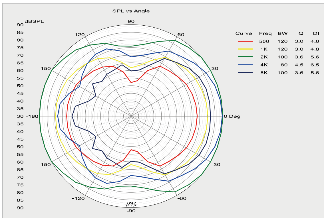
Круговая диаграмма направленности громкоговорителя LPA-06CL20 (цвет черный)
